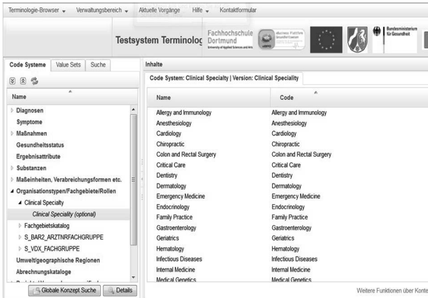
Abb. 3 Terminologiebrowser Bildschirmansatz
