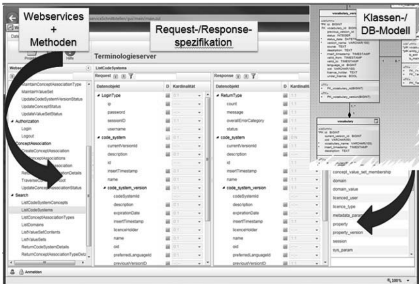
Abb. 2 Implementiertes Tool für den Dienstzuschnitt
